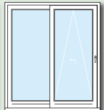
Hebeschiebekipp-Tür
